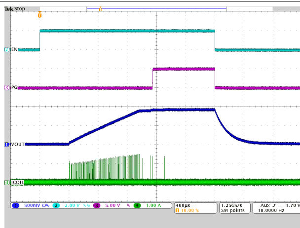
图 9-17. PSM Operation
