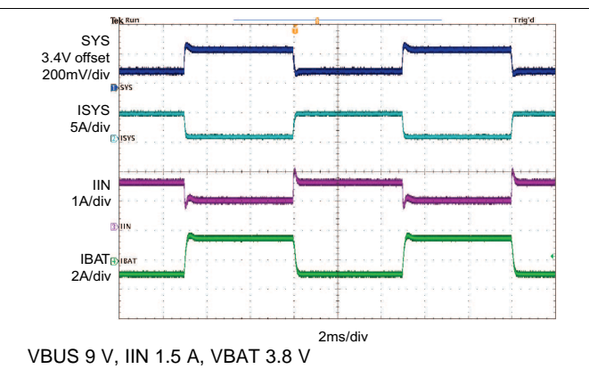
图 41. Charge Disable
