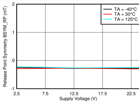
图 7-73. B_{SYM\_RP(XY)} vs. V_{CC}
