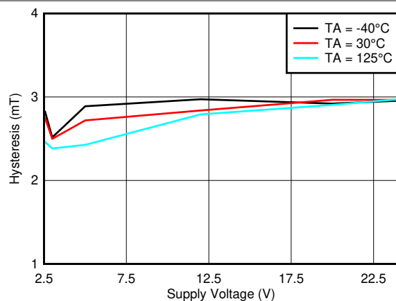
图 7-11. Hysteresis_X vs. V_{CC}
