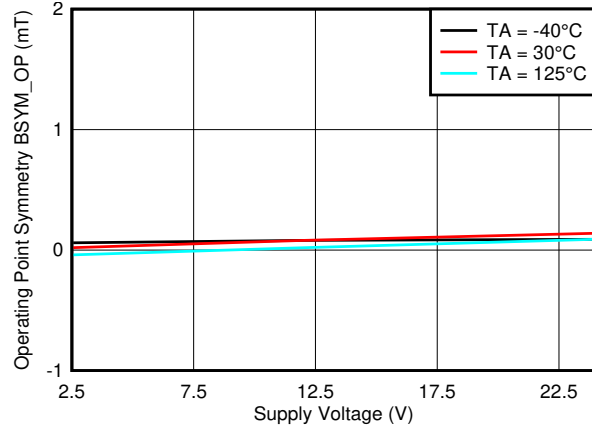
图 7-63. B_{SYM\_OP(ZX)} vs. V_{CC}
