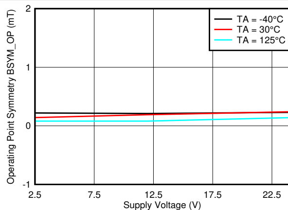
图 7-67. B_{SYM\_OP(ZY)} vs. V_{CC}
