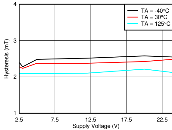
图 7-5. Hysteresis_Z vs. V CC
