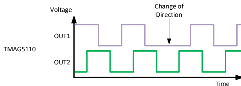
图 9-2. TMAG5110-Q1 Output Response
