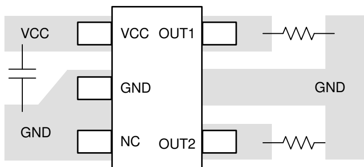
图 11-1. Layout Example
