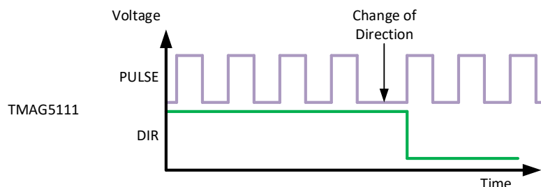
图 9-3. TMAG5111-Q1 Output Response
