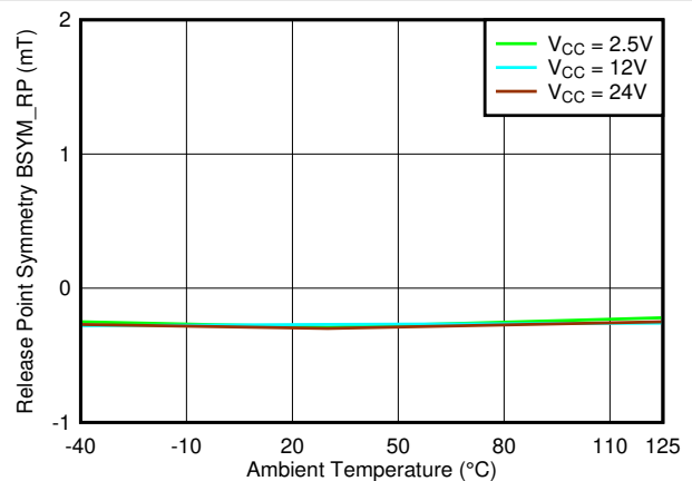
图 7-74. B_{SYM\_RP(XY)} vs. Temperature
