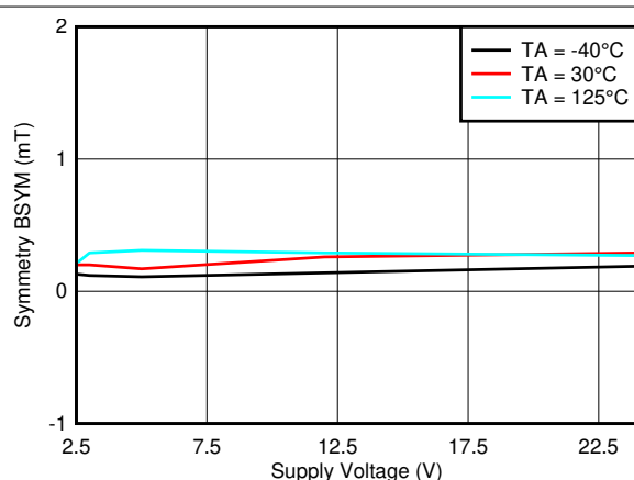
图 7-23. B_{SYM(y)} vs. V_{CC}
