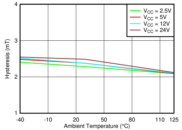
图 7-6. Hysteresis_Z vs. Temperature
