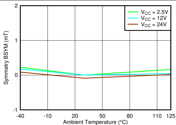
图 7-62. B_{SYM(Y)} vs. Temperature
