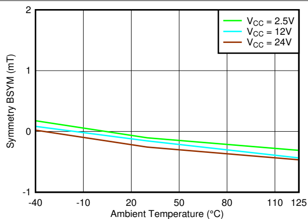
图 7-60. B_{SYM(X)} vs. Temperature
