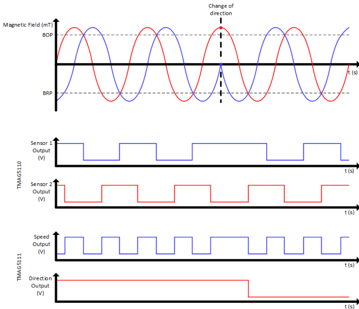
图 8-3. TMAG511x-Q1 Output Behavior
