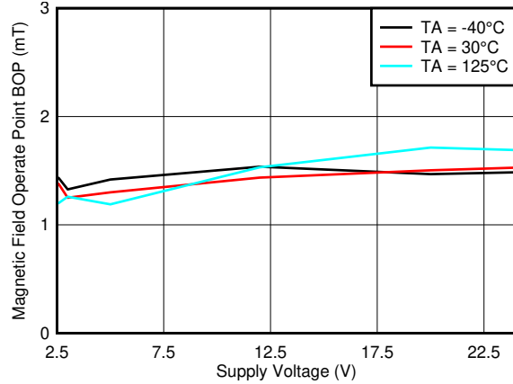
图 7-7. B_{OP\_X} Threshold vs. V_{CC}
