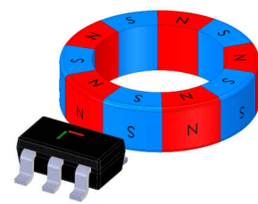
图 8-6. XY Outer Edge 2
