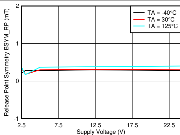
图 7-31. B_{SYM\_RP(ZY)} vs. V_{CC}
