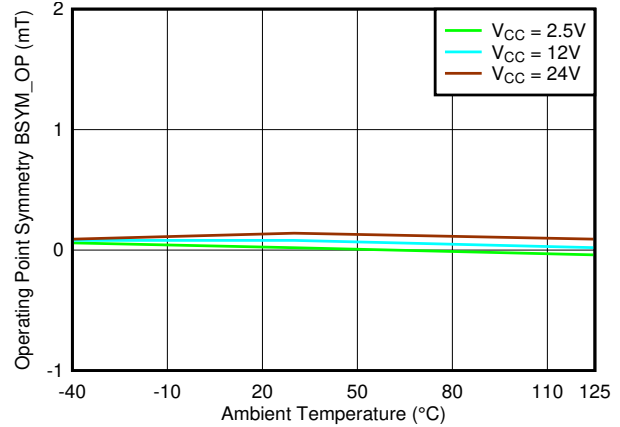
图 7-64. B_{SYM\_OP(ZX)} vs. Temperature
