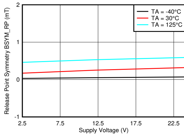
图 7-65. B_{SYM\_RP(ZX)} vs. V_{CC}
