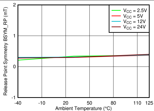
图 7-32. B_{SYM\_RP(ZY)} vs. Temperature
