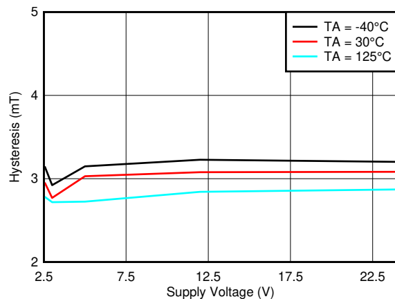
图 7-17. Hysteresis_Y vs. V CC
