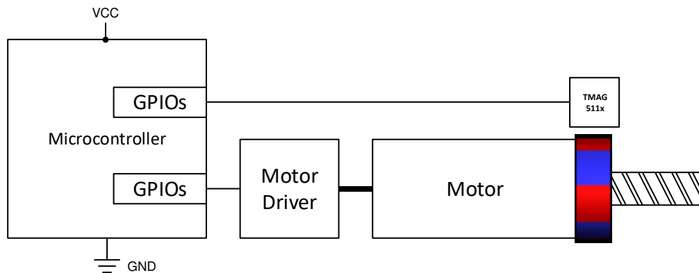
图 9-1. Incremental Encoding
