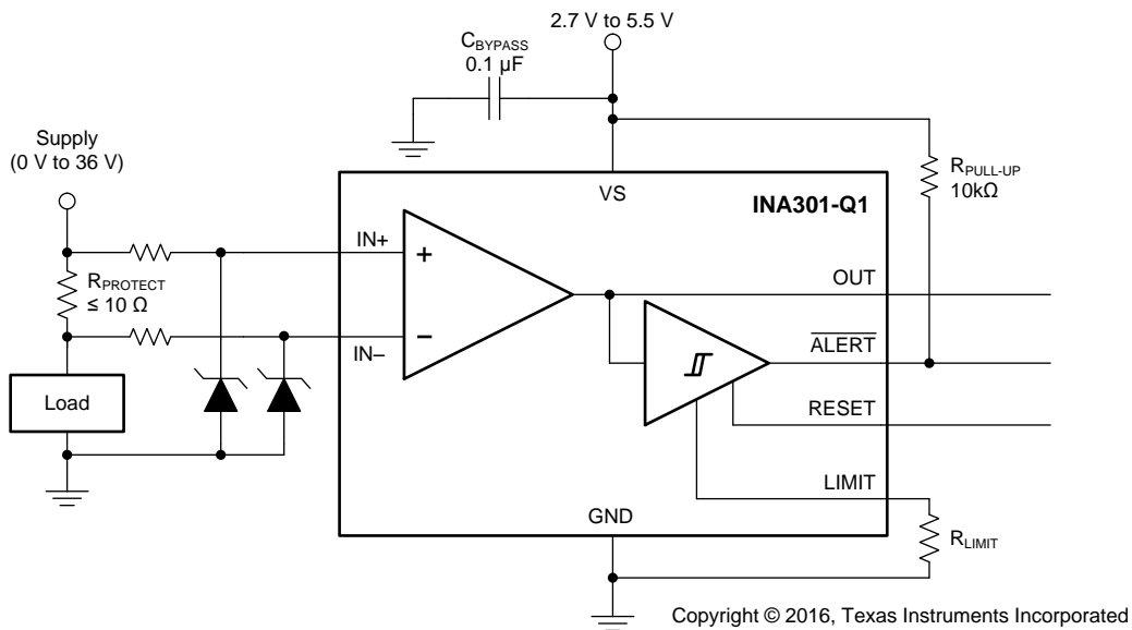
图 41. Transient Protection
