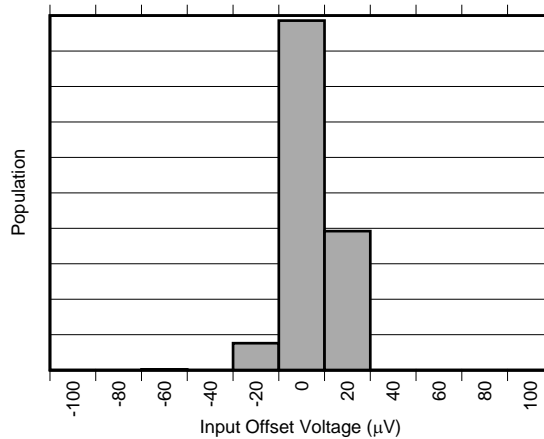
图 2. Input Offset Voltage Distribution (INA301A2-Q1)
