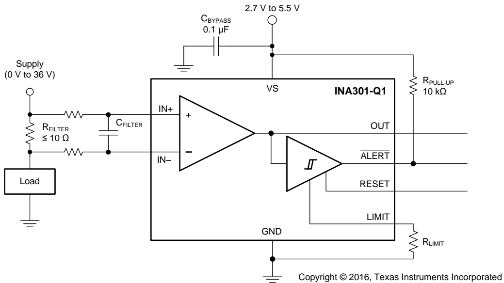
图 39. Input Filter
