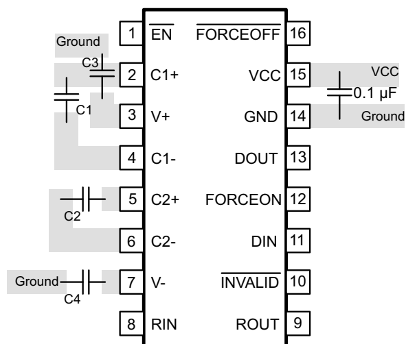
图 10-1. Layout Diagram
