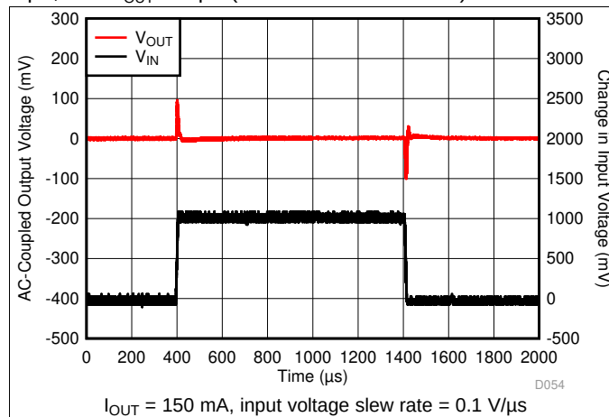
图 19. V_{IN} Transient
