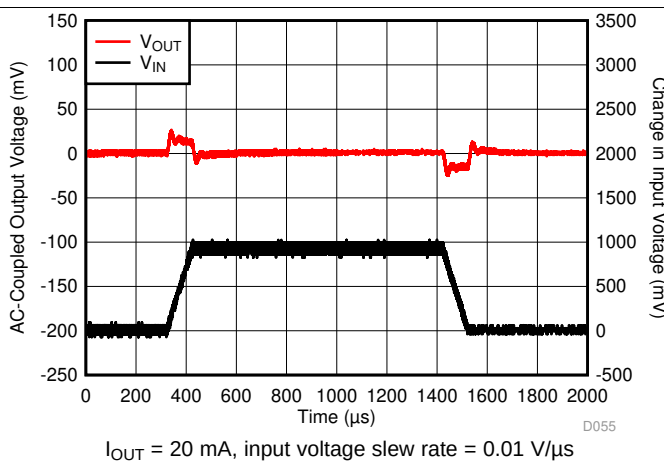
图 20. V_{IN} Transient
