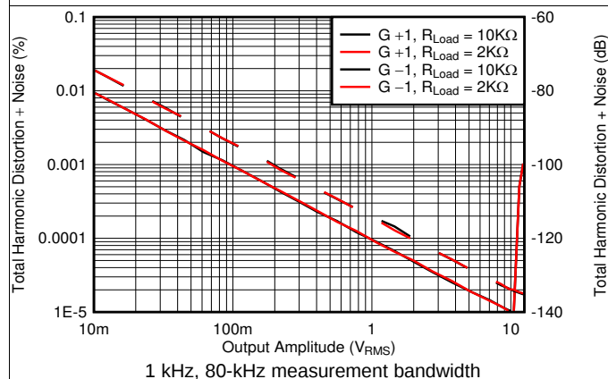
图 11. THD+N vs Output Amplitude
