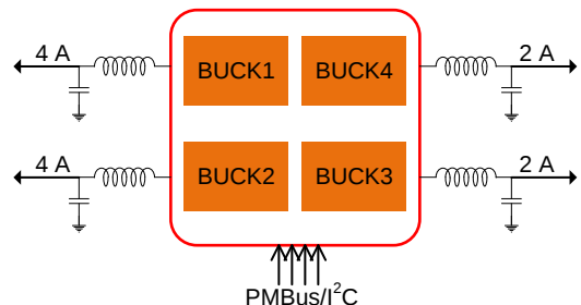
简化电路原理图
