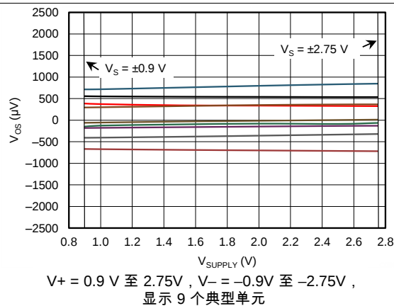
Figure 5. 失调电压与电源间的关系
