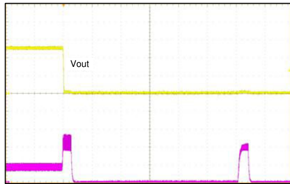
图 8-7. Hiccup Operation
