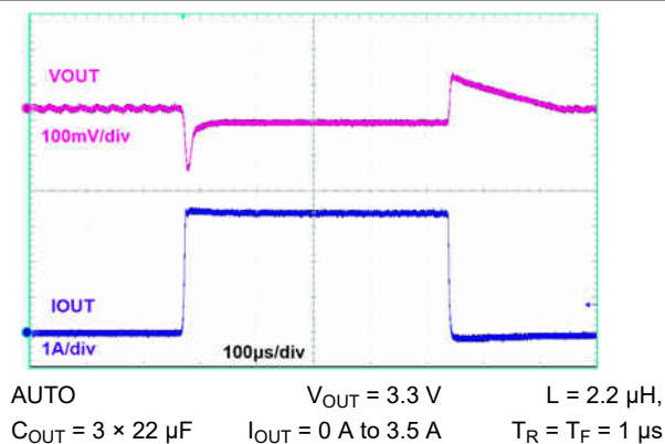
图 9-30. Load Transient
