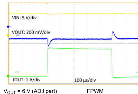
图 9-38. Load Transient
