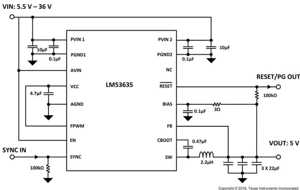
图 9-4. Fixed 5-V, 3.5-A Output Power Supply
