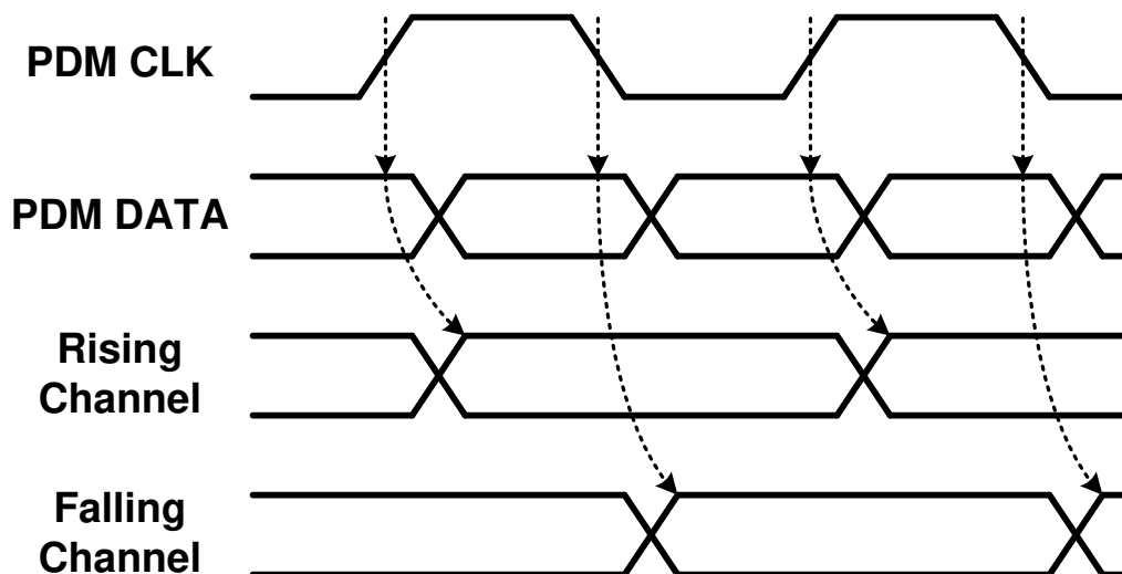
图 8-11. PDM Waveform
