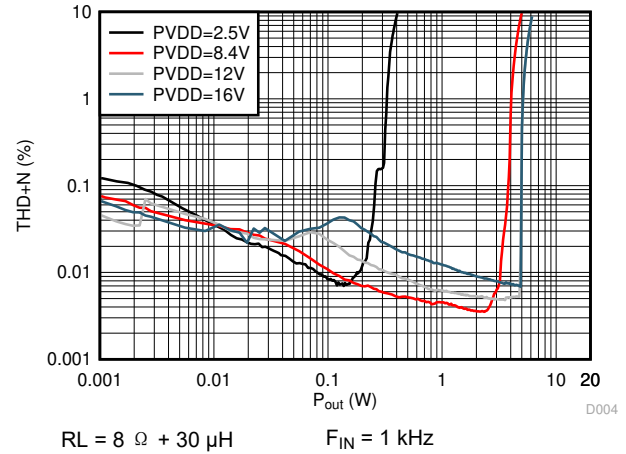
图 6-10. THD+N vs Output Power
