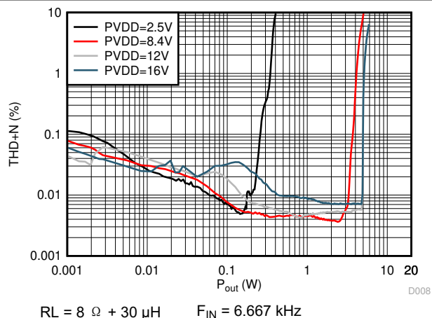
图 6-16. THD+N vs Output Power
