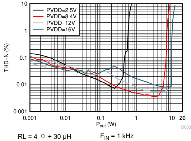
图 6-9. THD+N vs Output Power
