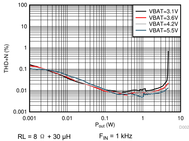
图 6-7. THD+N vs Output Power (DSBGA Package)
