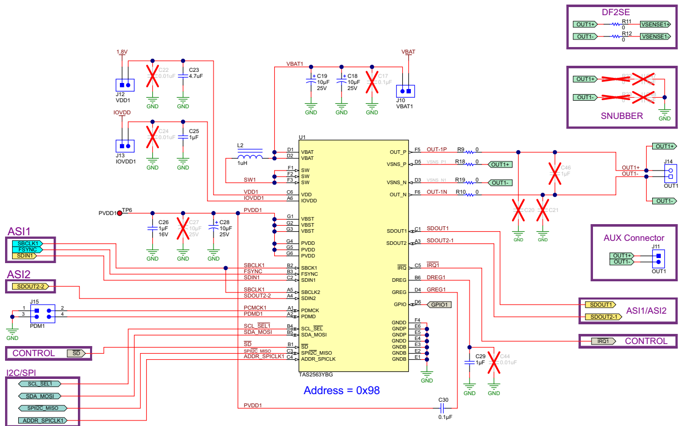
图 7-1. TAS2563 Circuit
