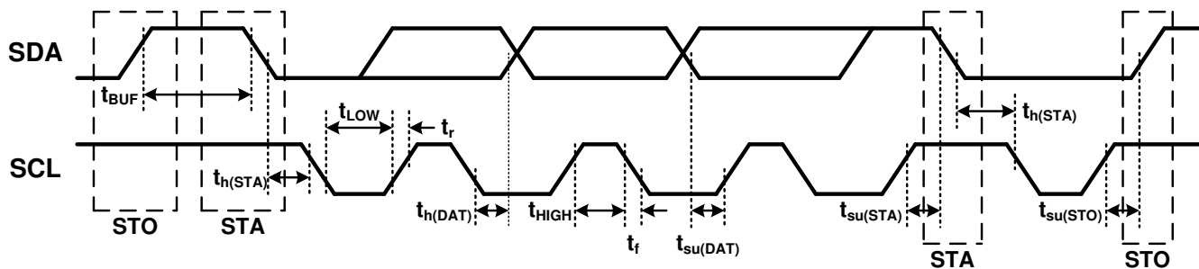
图 6-1. I²C Timing Diagram
