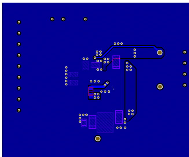
图 11-8. QFN Package Bottom Layer
