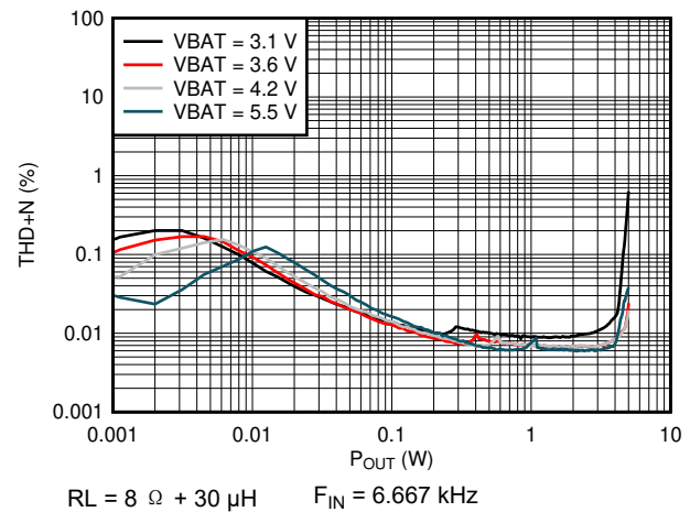
图 6-14. THD+N vs Output Power (QFN Package)
