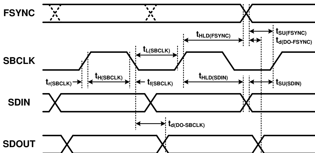
图 6-2. TDM Timing Diagram
