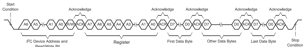
图 8-7. Multi-Byte Write Transfer
