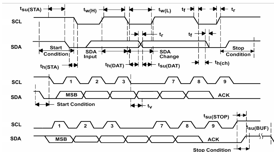
图 6-1. I²C Timing
