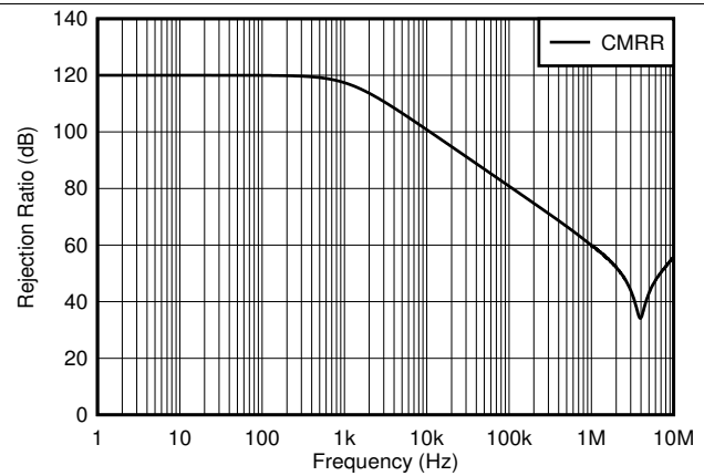
图 20. CMRR vs Frequency
