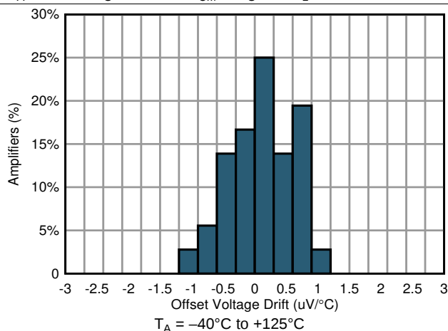
图 7. Offset Voltage Drift
