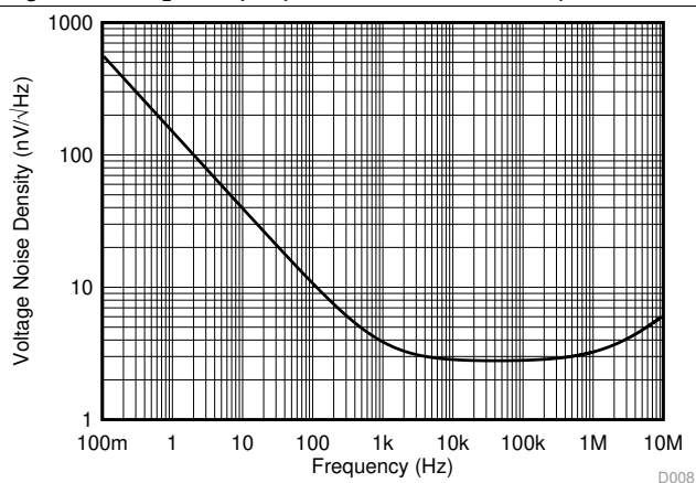
图 8. Input Voltage Noise Spectral Density
