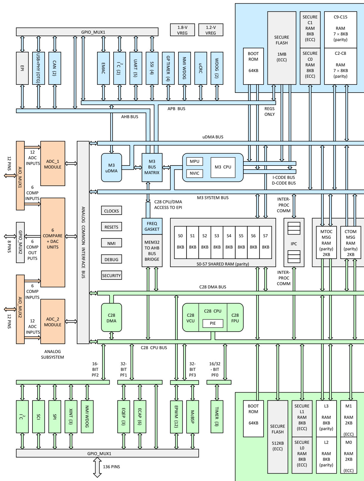
图 1-1. 功能框图
