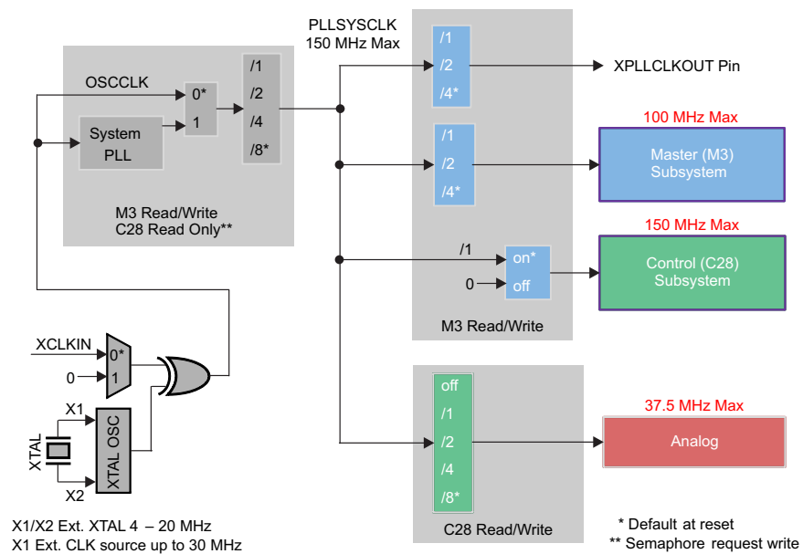
图 6-11. System Clock/PLL
