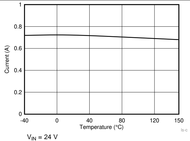
图 5. Low Side Current Limit
