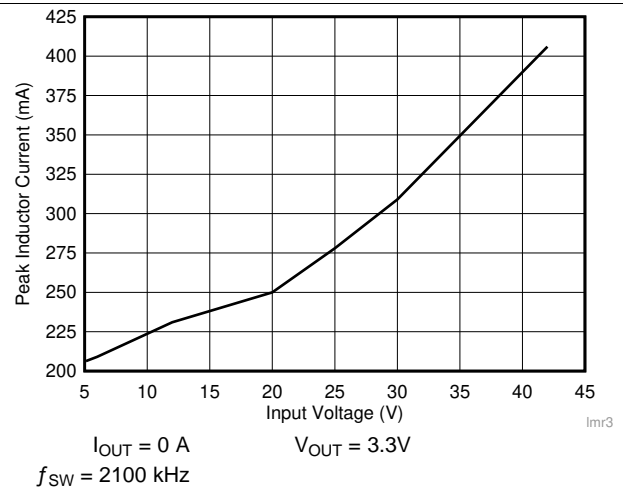
图 7. I PEAK-MIN
