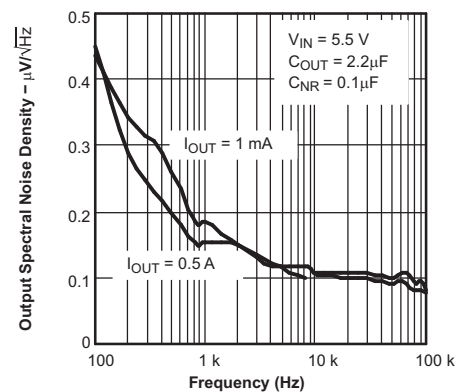
TPS79530 与频率
