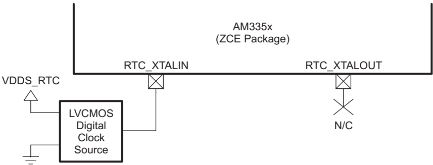
图 6-15. OSC1 (ZCE 封装) LVC MOS 电路原理图
