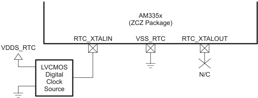
图 6-16. OSC1 (ZCZ 封装) LVC MOS 电路原理图
