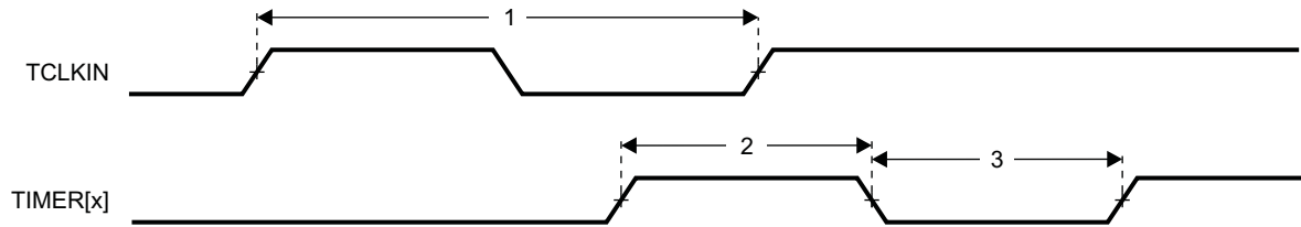
图 7-2. Timer Timing
