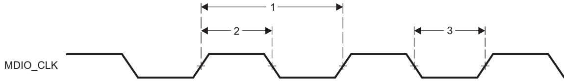
图 7-4. MDIO_CLK Timing
