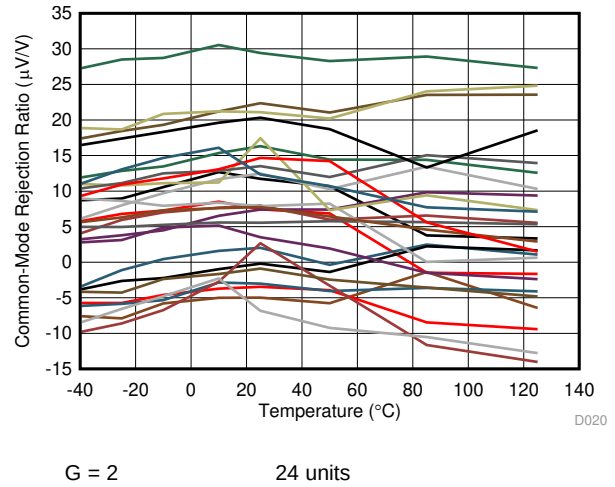
图 20. CMRR vs Temperature
