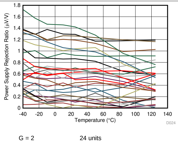
图 24. PSRR vs Temperature
