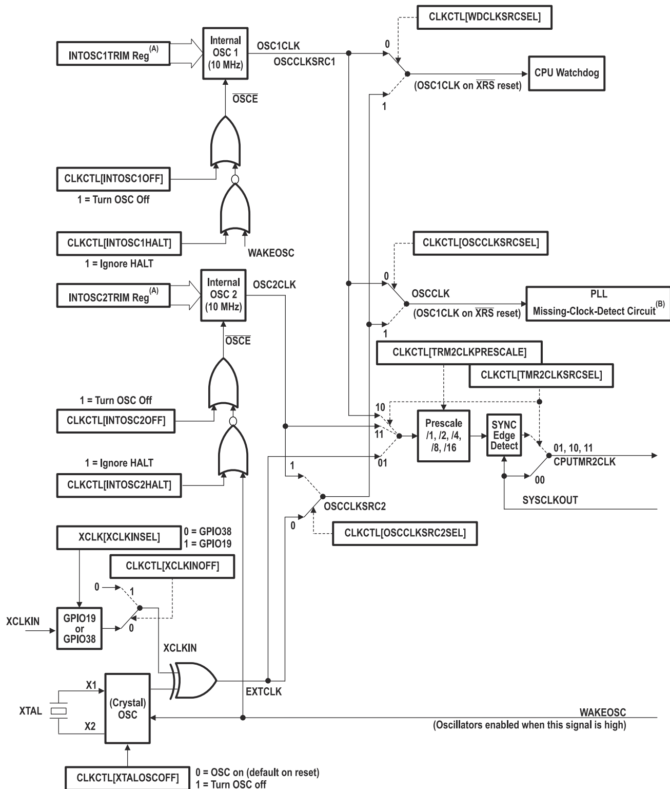
图 8-7. Clock Tree
