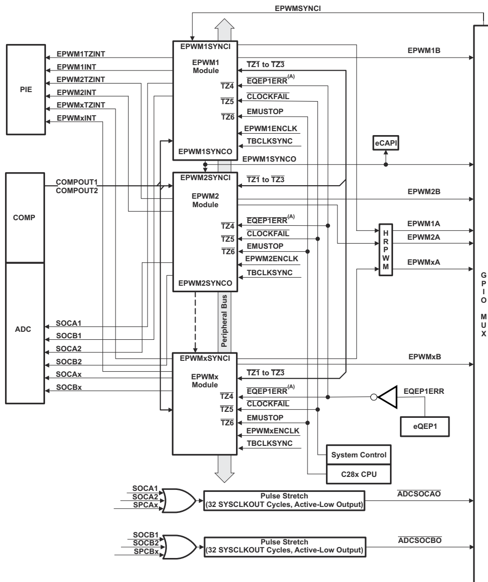
图 8-38. ePWM
