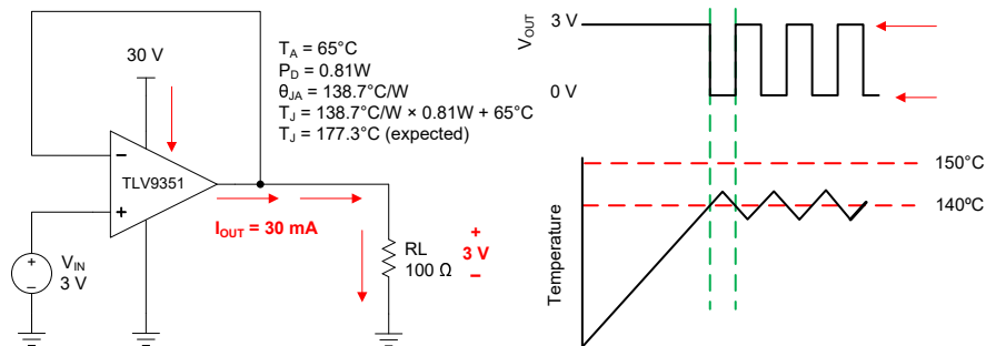
图 7-4. Thermal Protection
