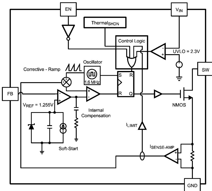
图 1：简化方框图
