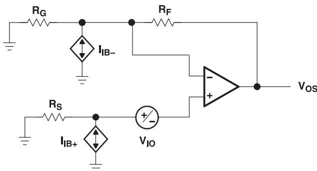
图 54. Output Offset Voltage Model
