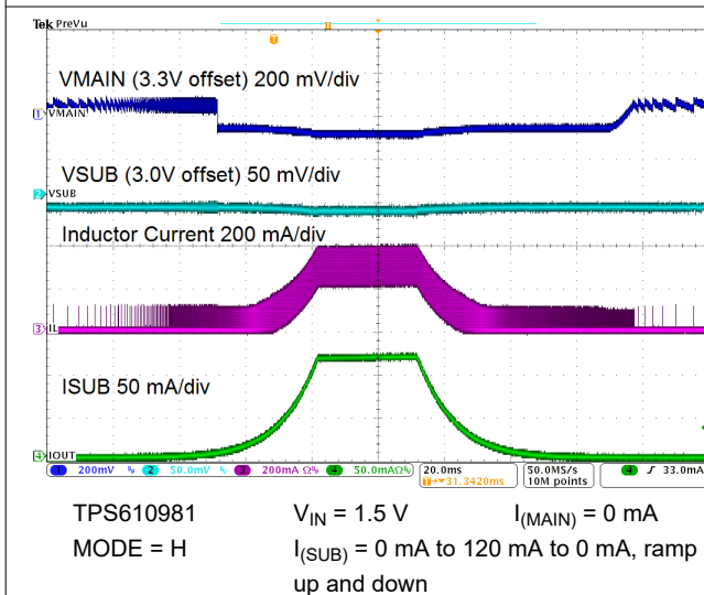
图 9-19. Load Regulation
