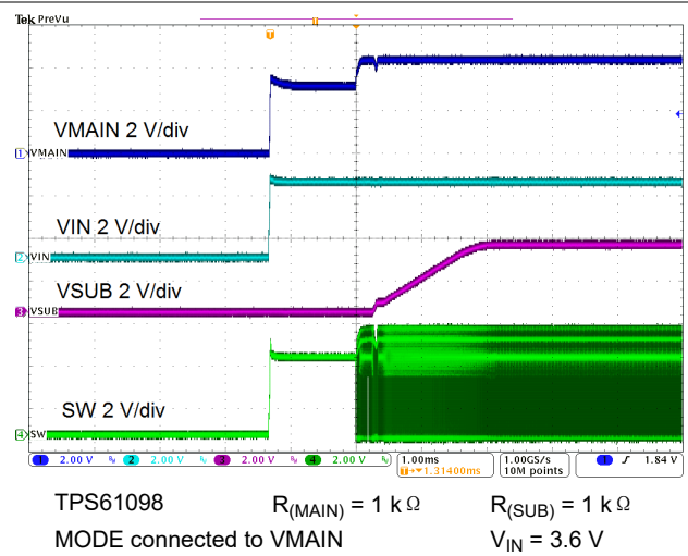
图 9-37. Startup
