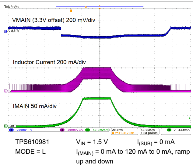
图 9-18. Load Regulation
