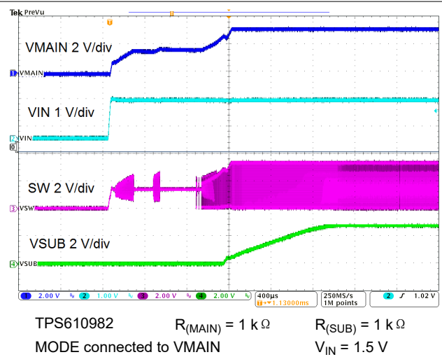
图 9-39. Startup
