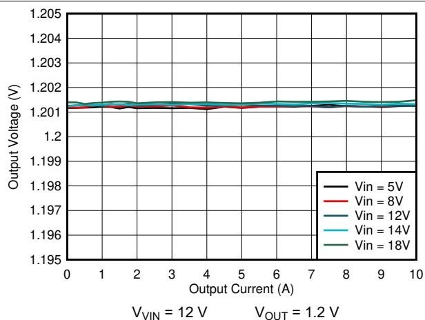
图 8-3. Load Regulation
