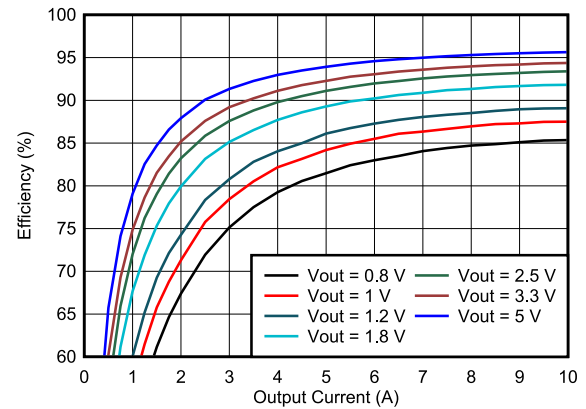
图 6-4. TPS546A24A Efficiency vs Output Current
