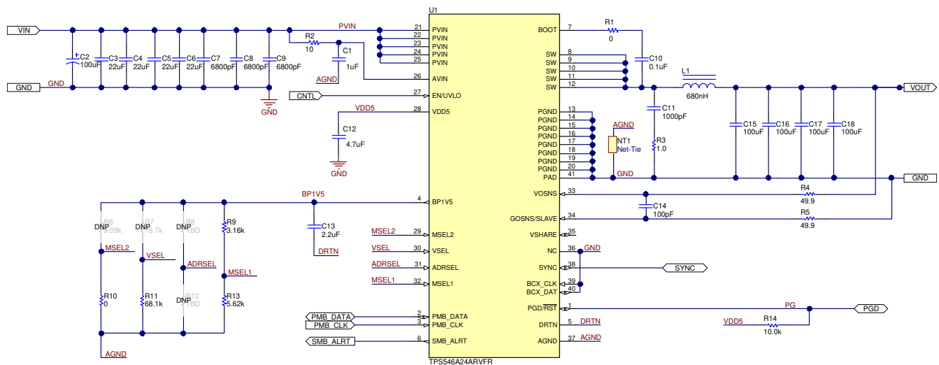
图 8-1. TPS546A24A Application
