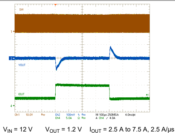
图 8-7. Load Transient Response
