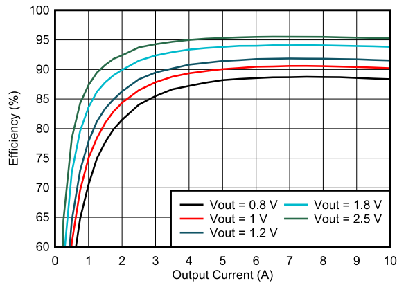
图 6-3. TPS546A24A Efficiency vs Output Current
