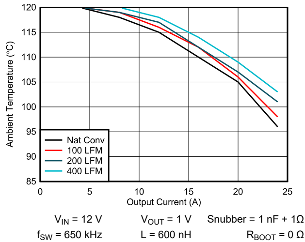
图 6-1. TPS546A24A Safe Operating Area
