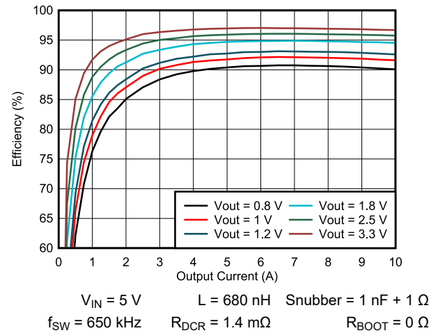
图 6-2. TPS546A24A Efficiency vs Output Current
