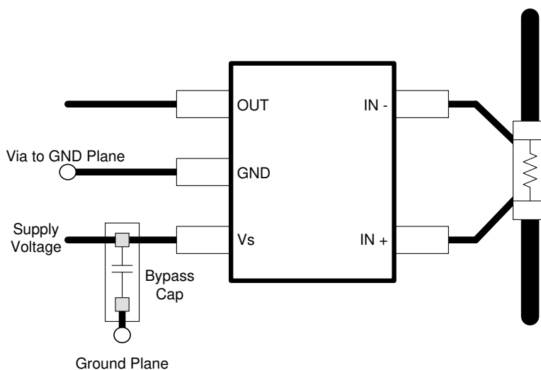
图 10-2. INA293B-Q1 Recommended Layout
