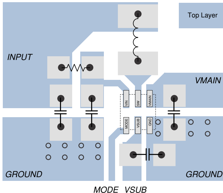
图 11-1. Layout
