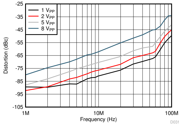
图 6-31. HD2 vs Output Voltage
