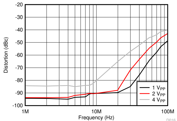
图 6-16. HD3 vs Output Voltage
