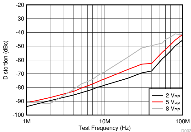
图 6-3. HD2 vs Frequency
