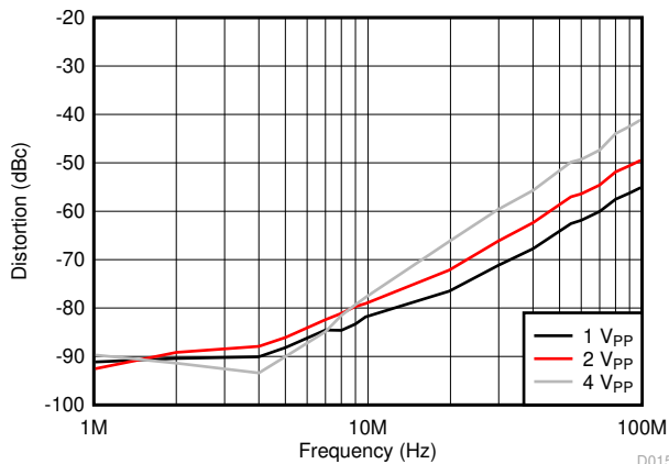
图 6-15. HD2 vs Output Voltage
