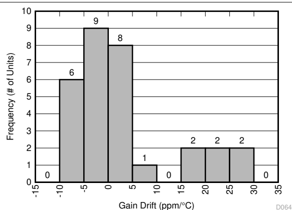
图 6-62. D2S Gain Drift Histogram
