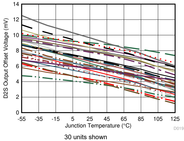
图 6-19. Output DC Offset Voltage vs Die Temperature
