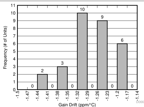
图 6-64. OPS Gain Drift Histogram
