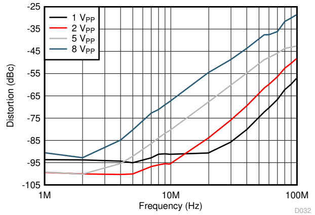
图 6-32. HD3 vs Output Voltage
