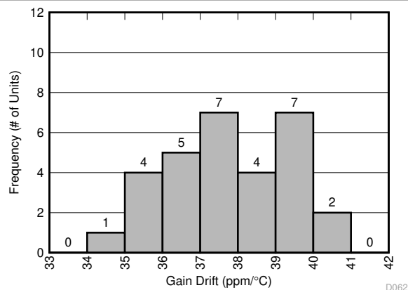
图 6-62. D2S Gain Drift Histogram
