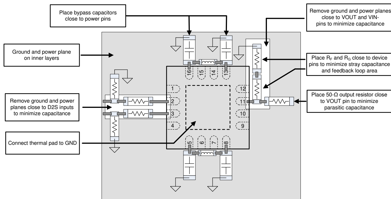
图 11-1. Layout Example
