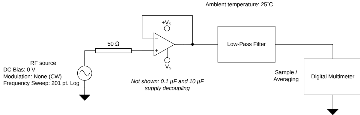
图 44. EMIRR IN+ 测试配置原理图
