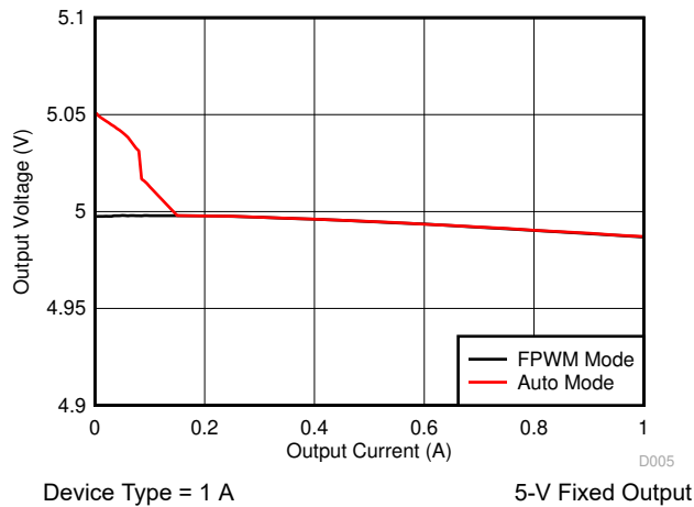
图 9-6. Load Regulation
