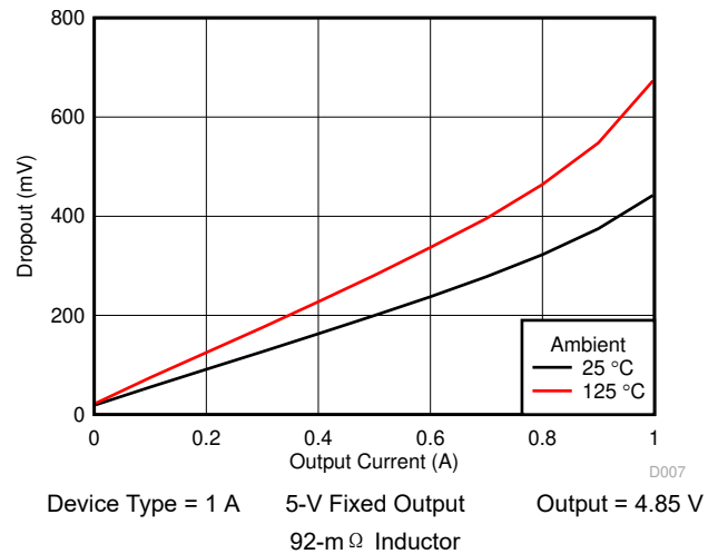
图 9-7. Dropout Voltage
