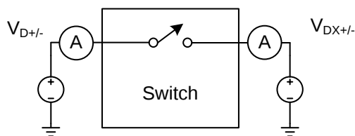
图 6. Off Leakage
