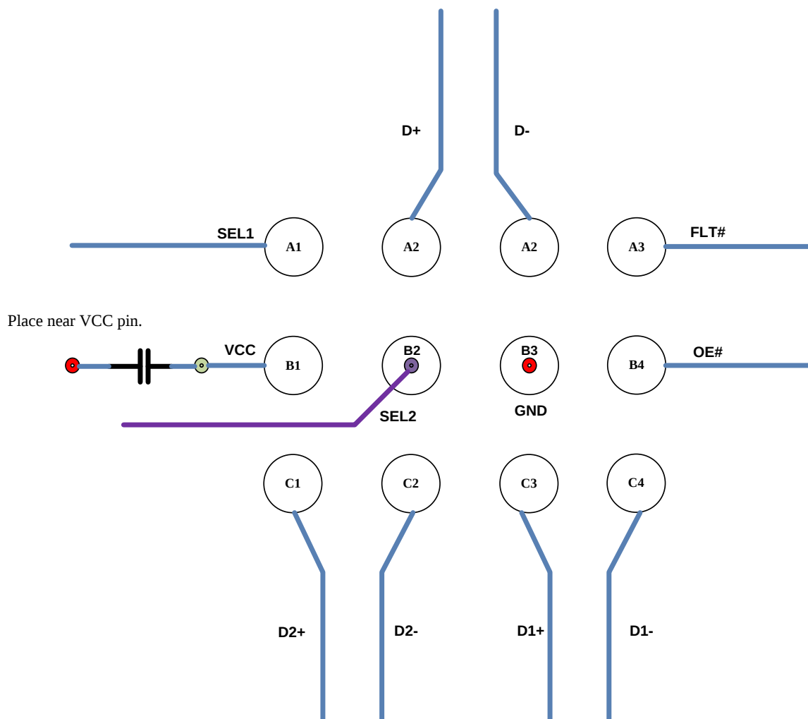
图 24. Layout Example
