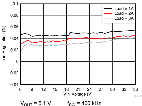
图 11-7. Line Regulation
