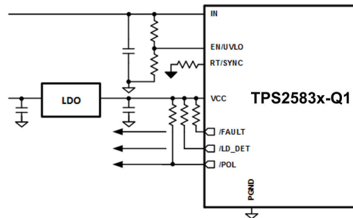
图 10-14. V_{\text{CONN}} Source Using External LDO
