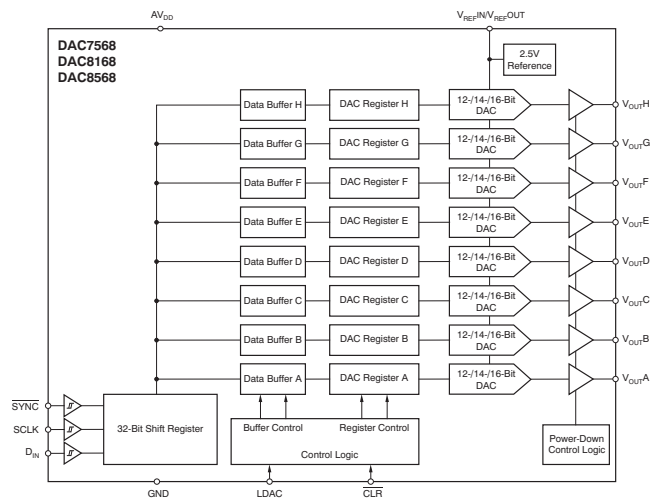
框图
