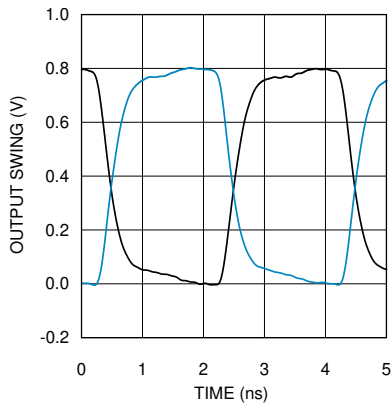
图 6-1. HCSL Output Swing at 250 MHz
