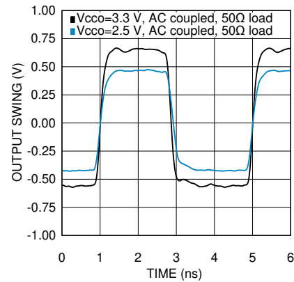
图 6-2. LVCMOS Output Swing at 250 MHz
