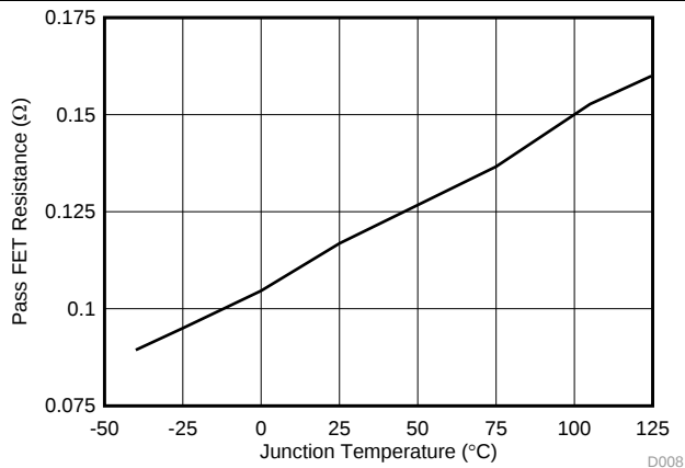
Figure 7. 导通 FET 电阻与温度间的关系 (TPS2372-4)
