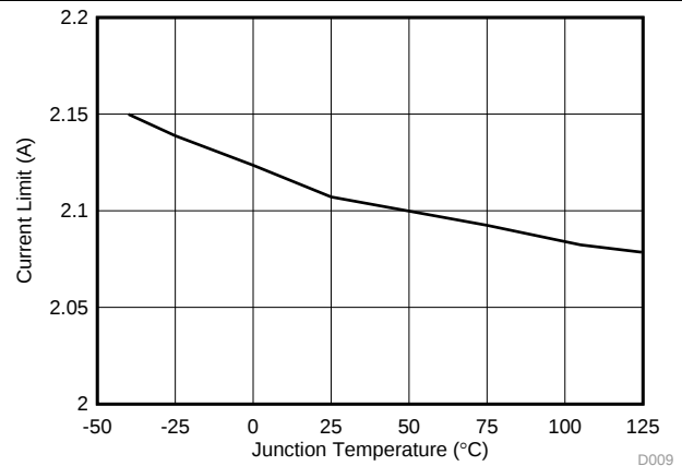
Figure 8. PoE 电流限制与温度间的关系 (TPS2372-4)
