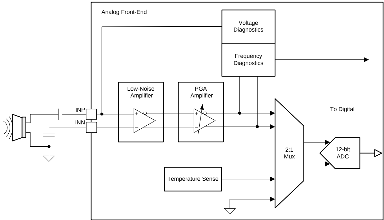
图 5. Analog Front-End
