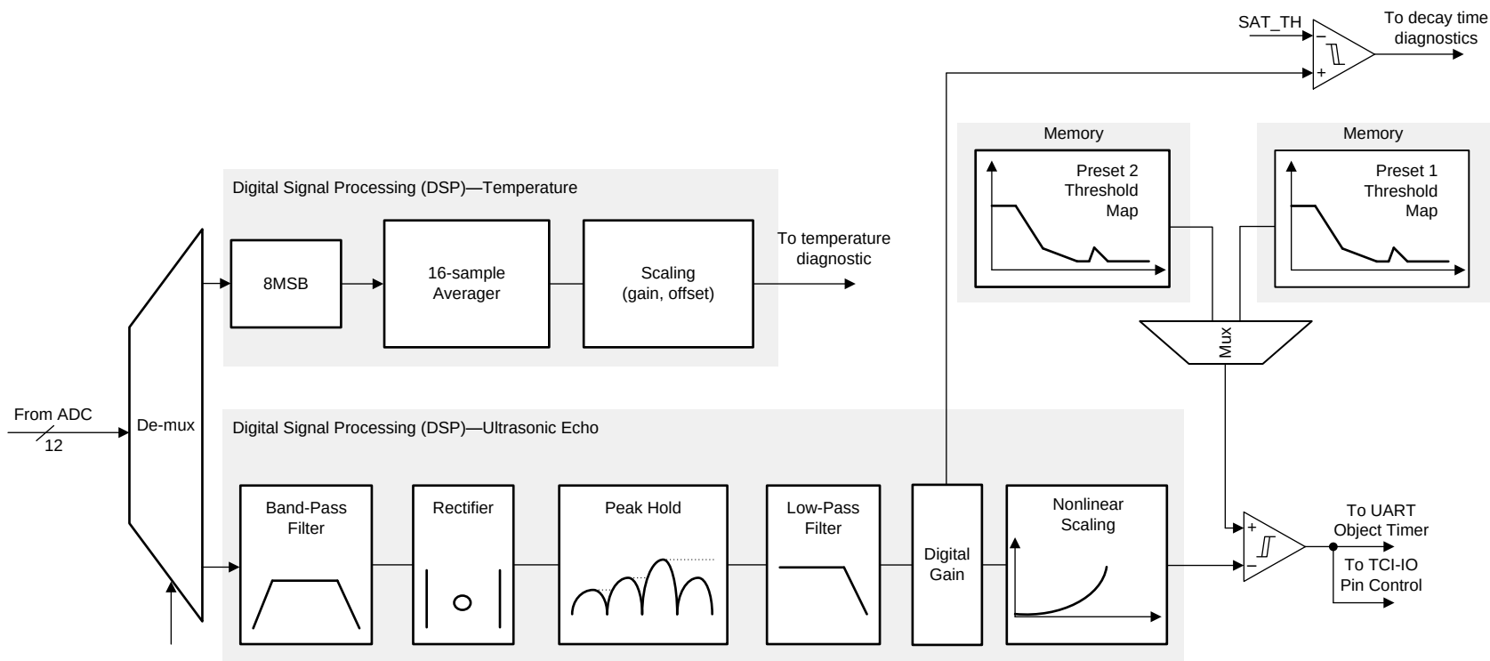
图 7. DSP Data-Path
