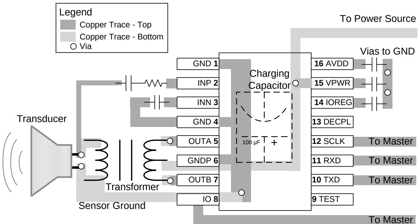
图 144. PGA460 Layout Example
