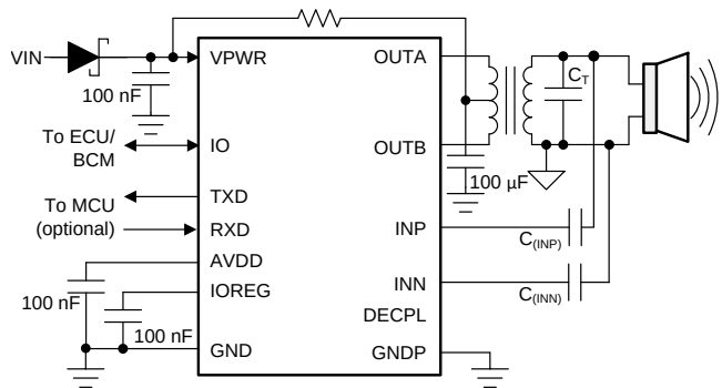
典型应用图（变压器驱动器）
