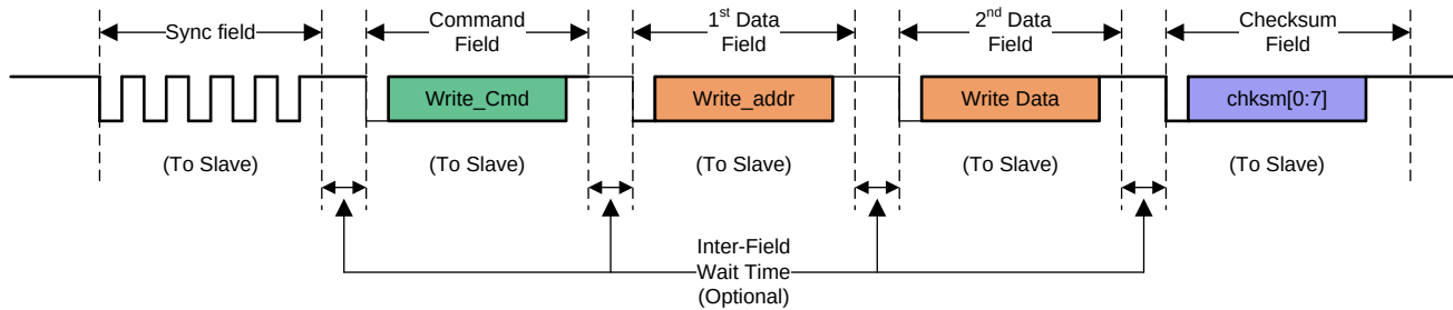
图 26. UART No-Response Example
