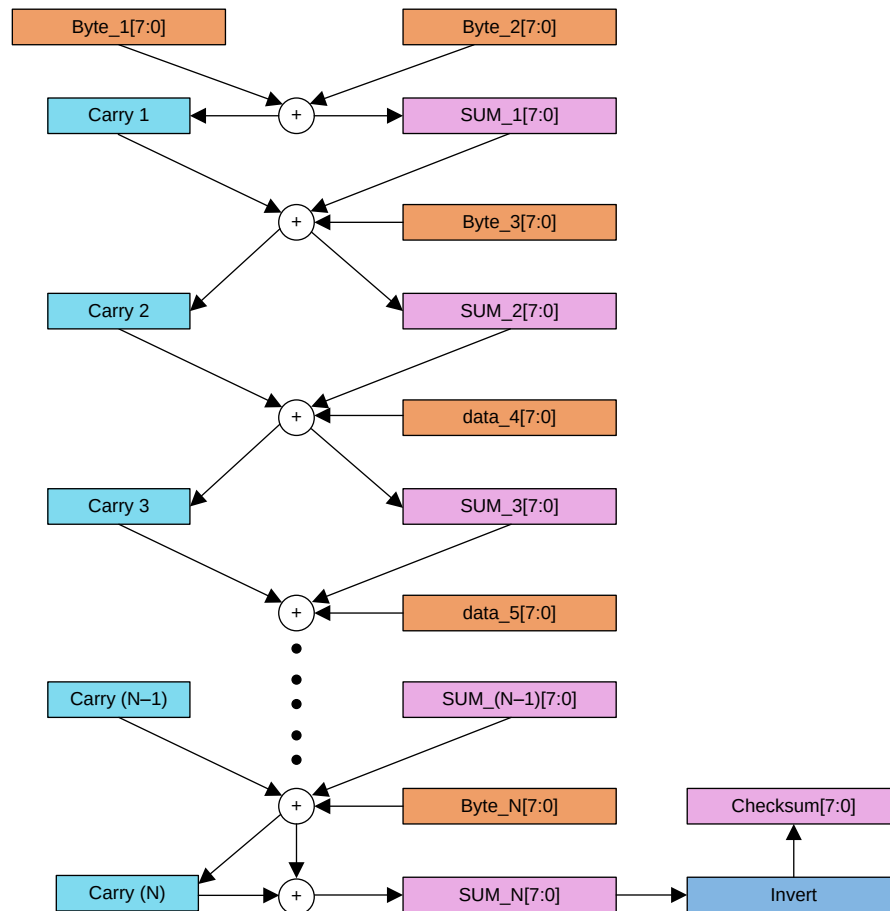
图 19. Checksum Calculation
