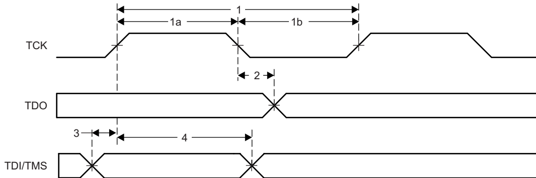
图 5-11. JTAG Timing
