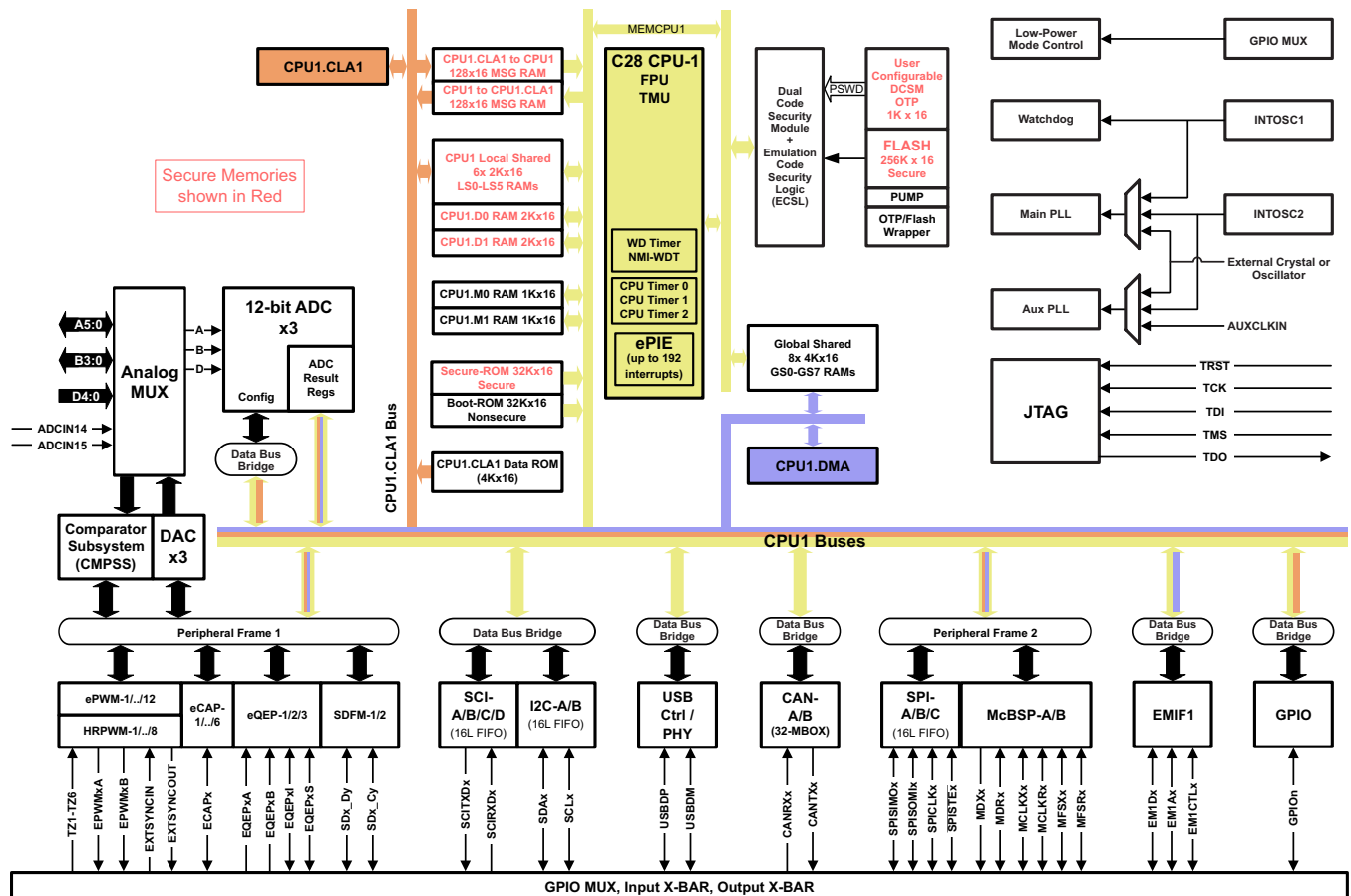
图 1-1. 功能方框图
