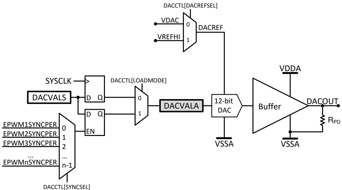
图 5-40. DAC Module Block Diagram
