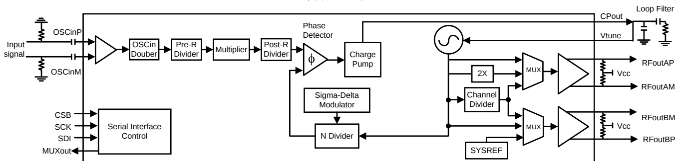
简化原理图
