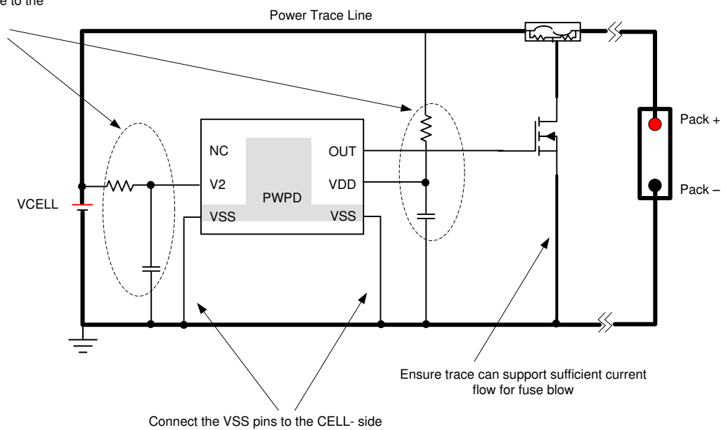
图 9-1. Layout Schematic
