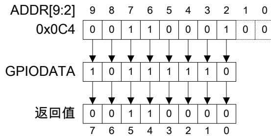
图 9-4. GPIODATA 读实例
