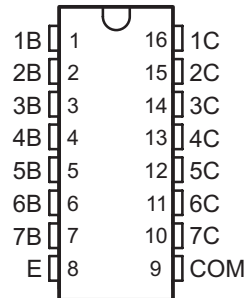
引脚功能
