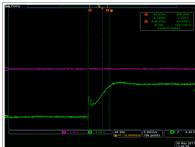
图 36. HO Rise Time
