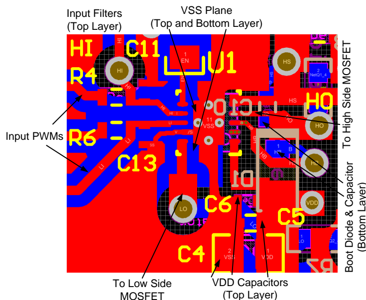
图 44. Layout Example
