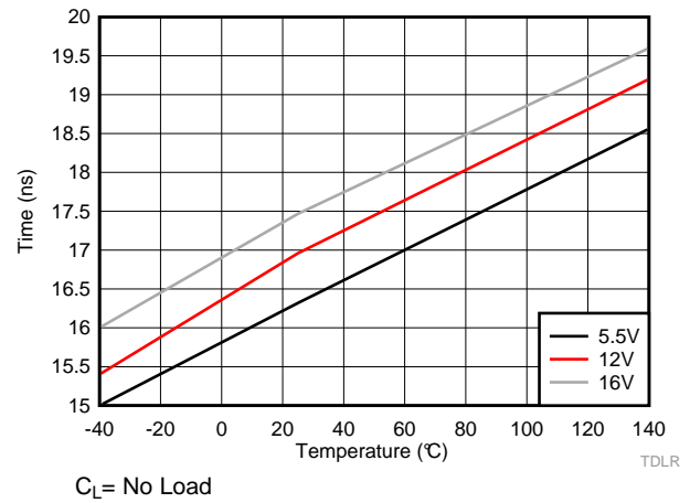
图 31. LO Rising Propagation Delay (TDLRR)
