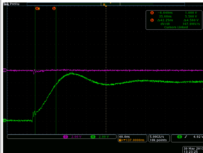
图 38. LO Rise Time
