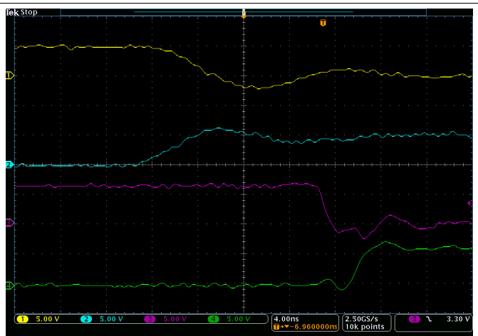
图 39. LO Fall Time
