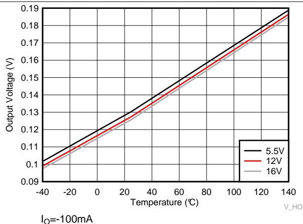
图 22. HO High Output Voltage ( V_{HOH} )
