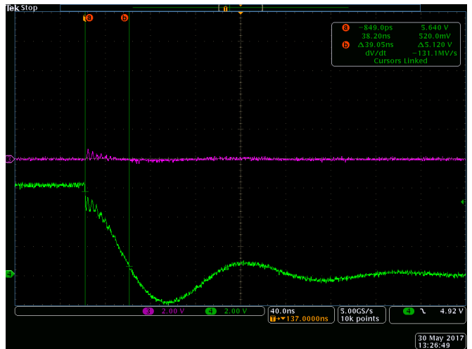
图 39. LO Fall Time
