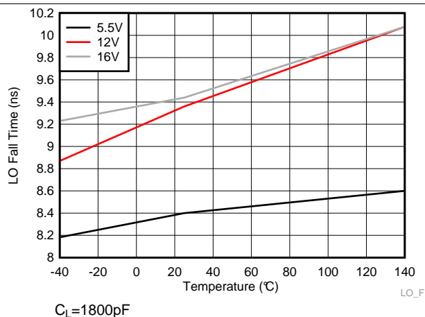
图 24. LO Fall Time
