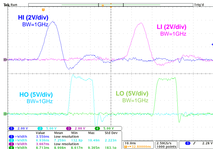
图 35. Input and Output Pulse Width
