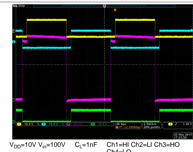
图 43. Input Negative Voltage
