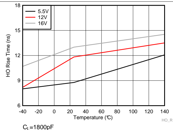
图 25. HO Rise Time
