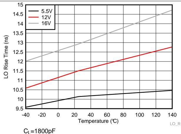
图 23. LO Rise Time
