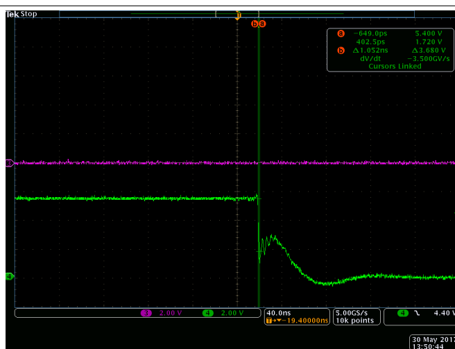
图 37. HO Fall Time
