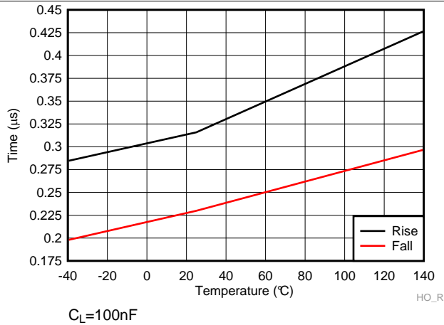
图 28. HO Rise & Fall Time
