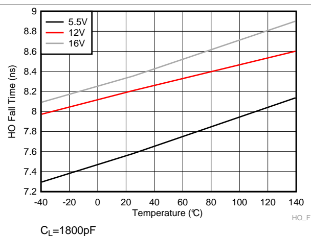
图 26. HO Fall Time
