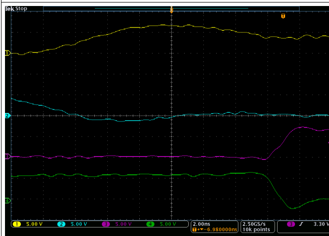
图 38. LO Rise Time
