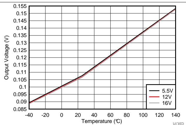
图 19. LO Low Output Voltage ( V_{LOL} )
