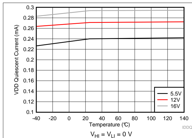
图 2. VDD Quiescent Current
