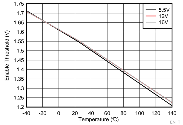
图 11. Enable Threshold
