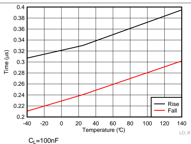
图 27. LO Rise & Fall Time
