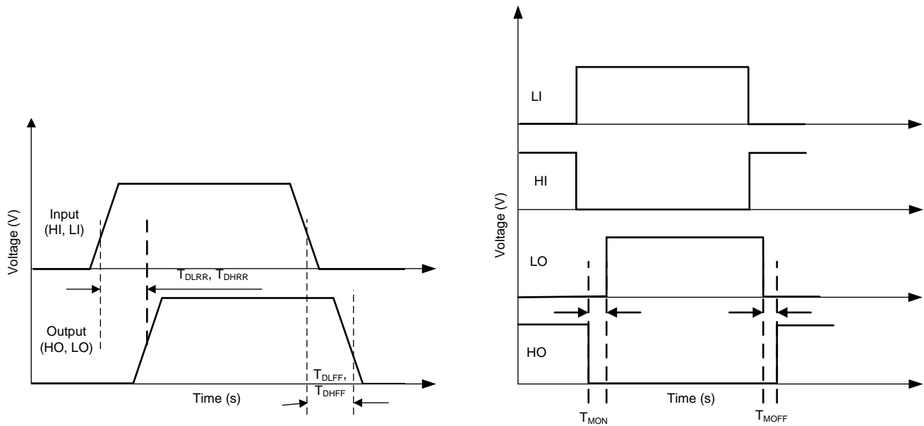
图 1. Timing Diagram
