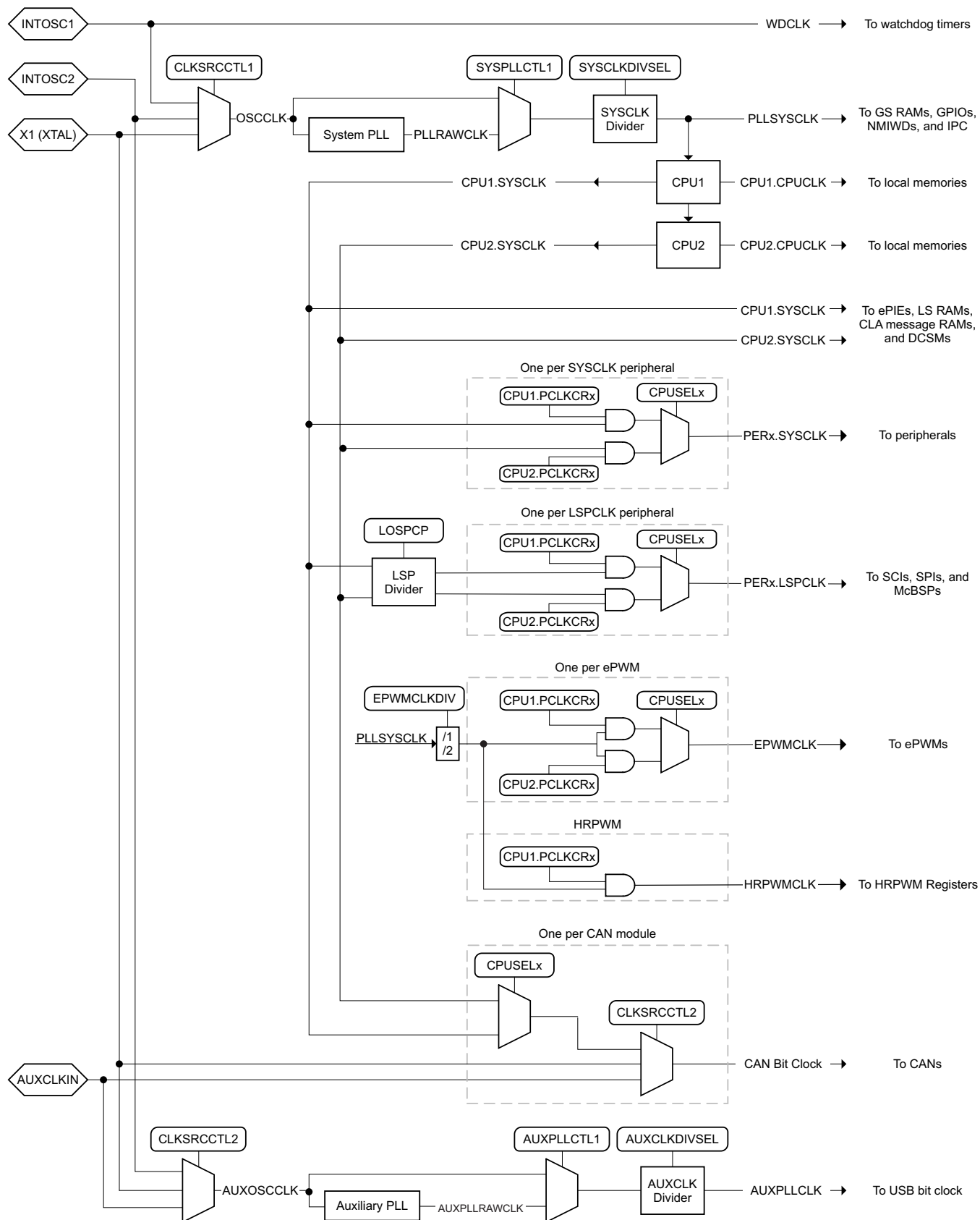
图 5-7. Clocking System
