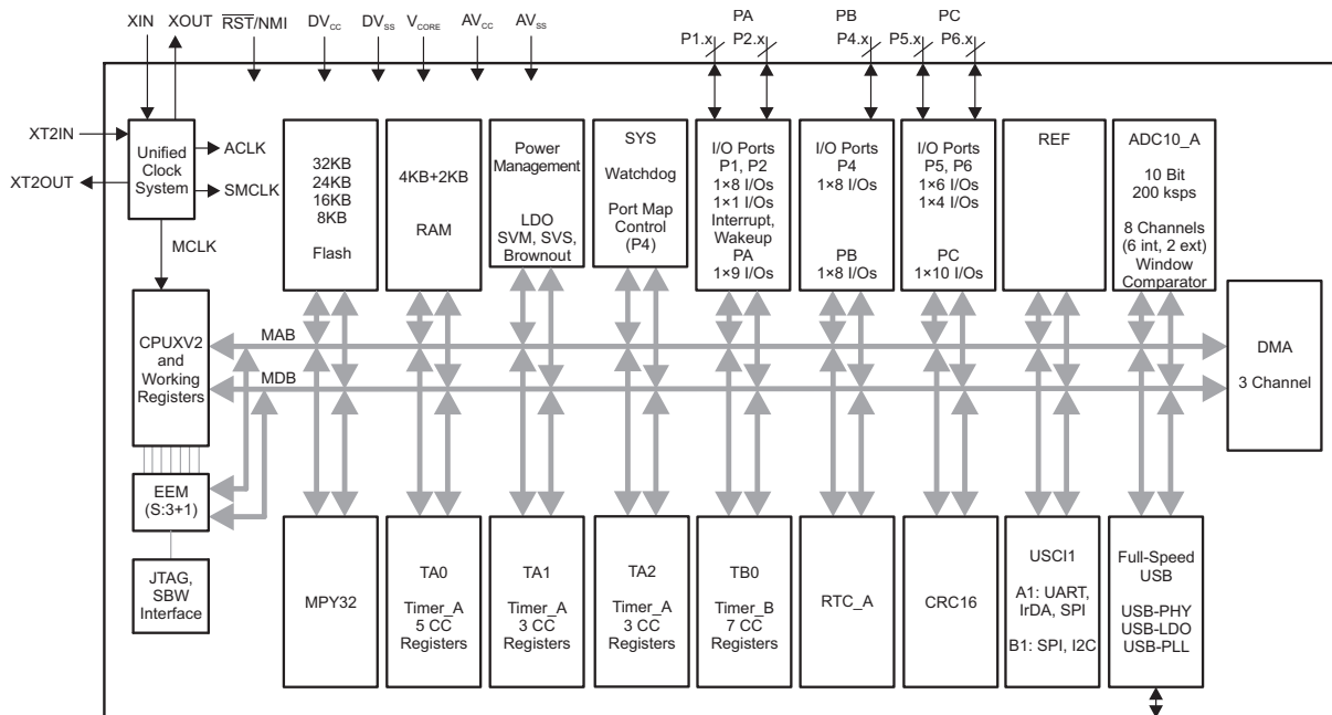
图 1-3. 功能方框图 - MSP430F5507IRGZ、MSP430F5506IRGZ、MSP430F5505IRGZ、MSP430F5504IRGZ、MSP430F5504IPT
