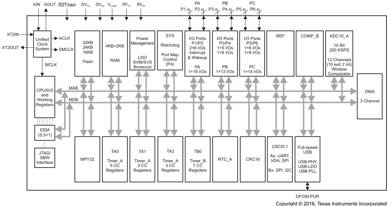
图 1-1. 功能方框图 - MSP430F5510IRGC、MSP430F5509IRGC、MSP430F5508IRGC、MSP430F5510IZQE、MSP430F5509IZQE、MSP430F5508IZQE
