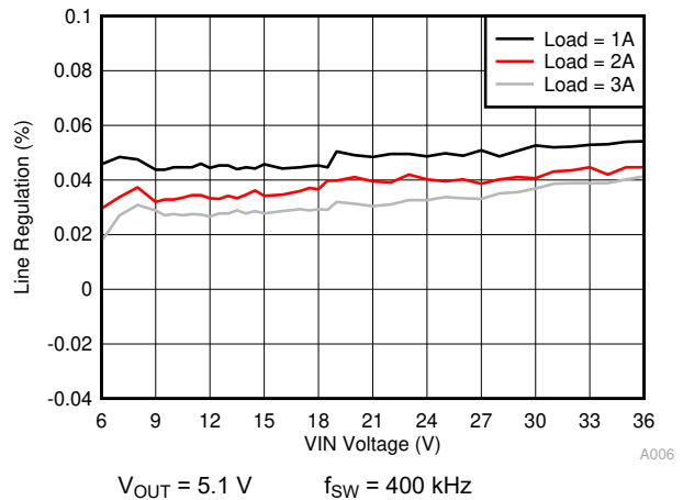
图 11-7. Line Regulation
