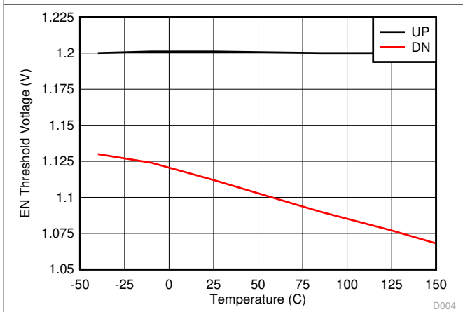
图 8-3. Precision Enable Threshold
