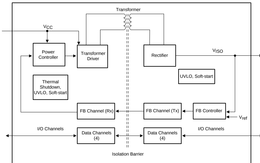
图 34. Block Diagram
