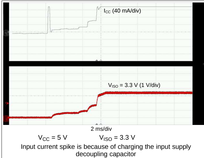
图 27. Soft Start at 120-mA Load
