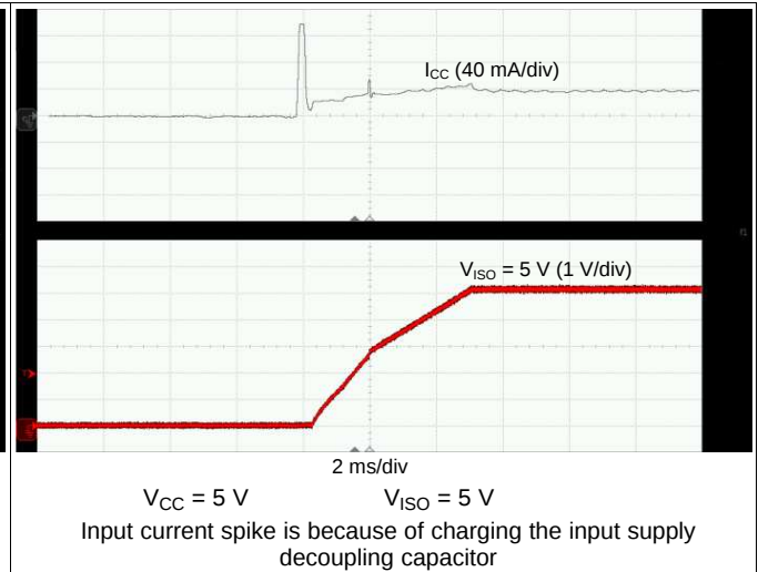
图 28. Soft Start at 10-mA Load
