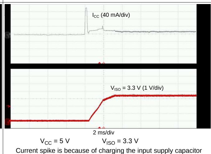
图 26. Soft Start at 10-mA Load
