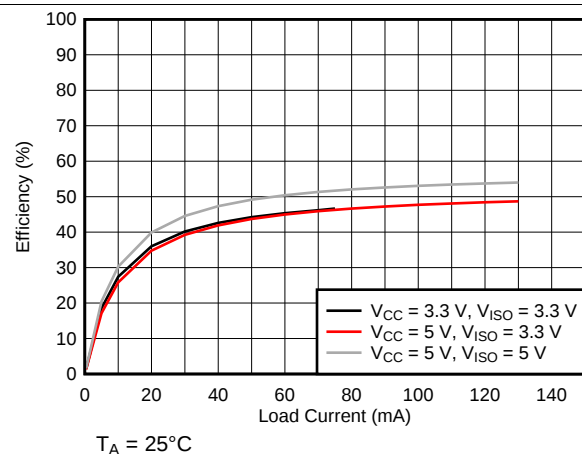
图 6. ISOW7841 Efficiency vs Load Current ( I_{ISO} )
