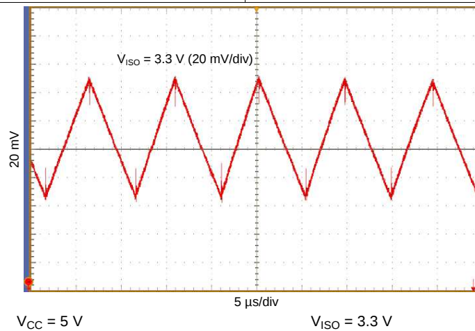
图 31. V_{ISO} Ripple Voltage at 130 mA
