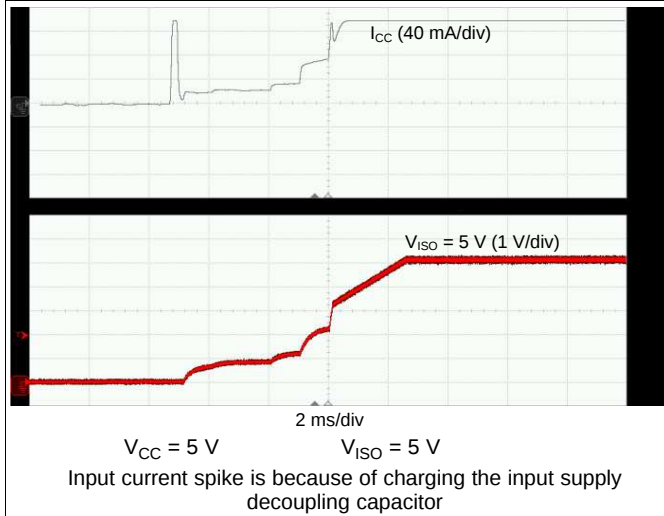
图 29. Soft Start at 130-mA Load
