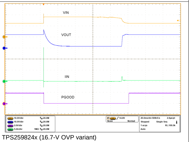
图 30. Overvoltage Protection
