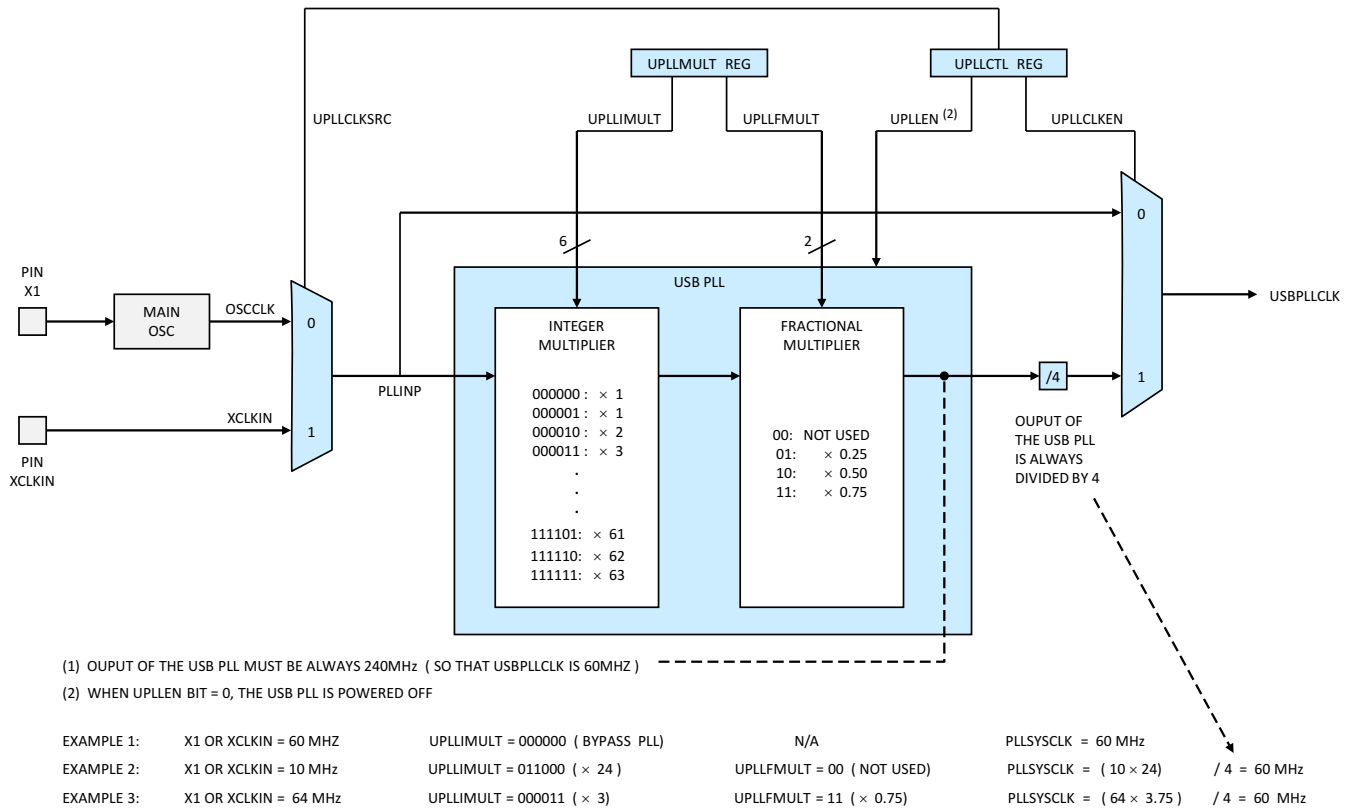
图 8-9. USB PLL
