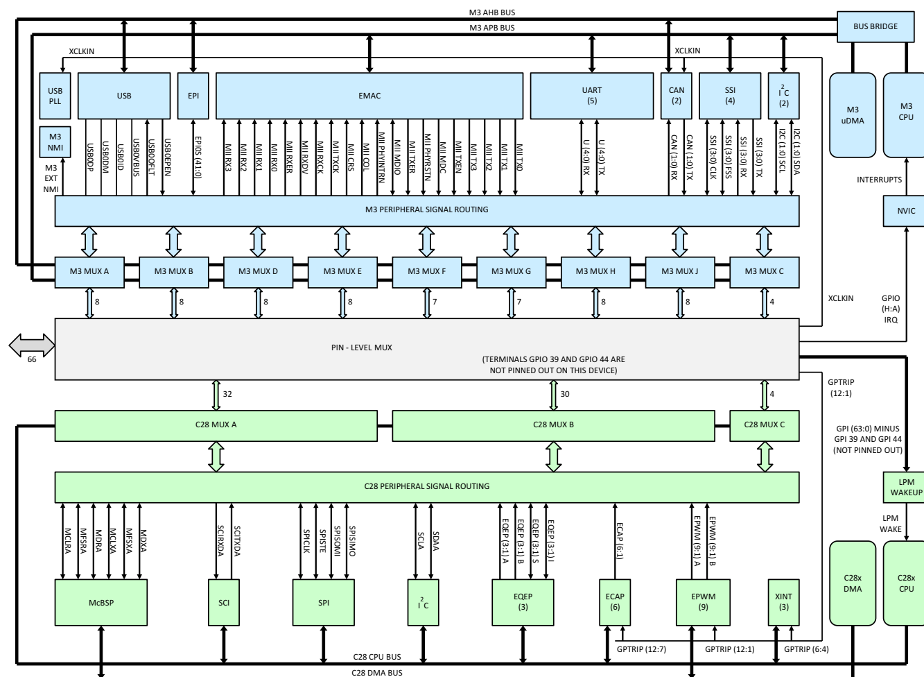
图 8-15. GPIO_MUX1 Block
