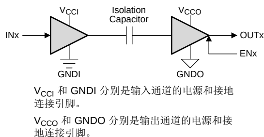
简化原理图
