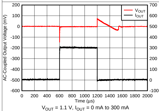
图 11. I_{OUT} Transient
