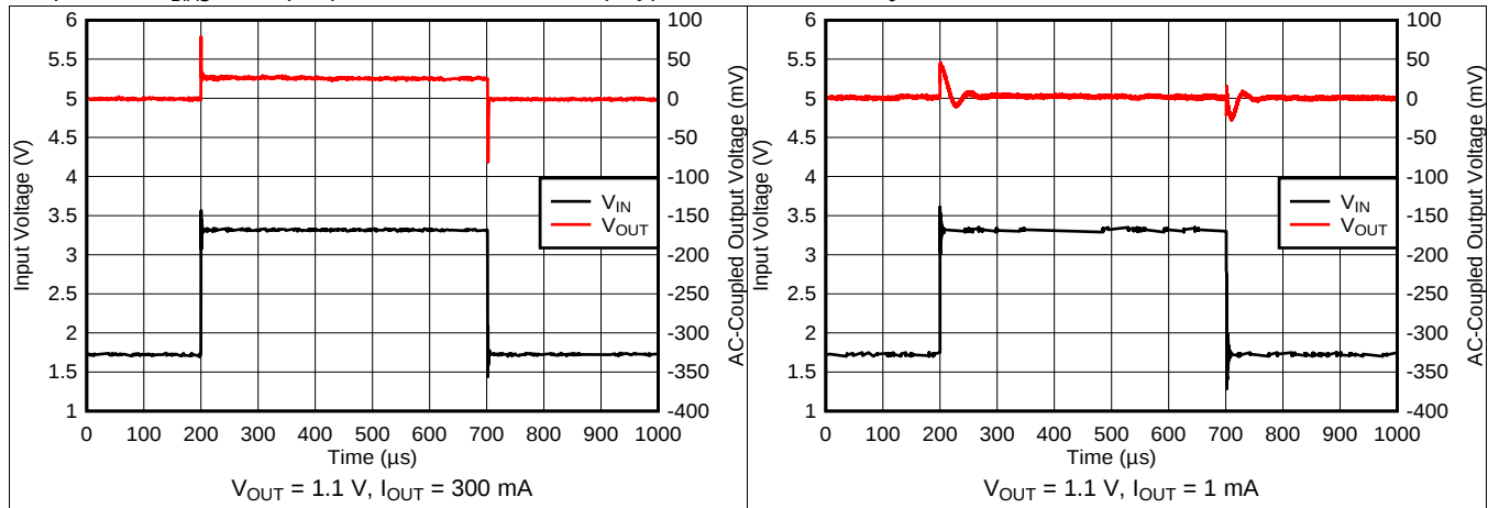
图 13. V_{IN} Transient
