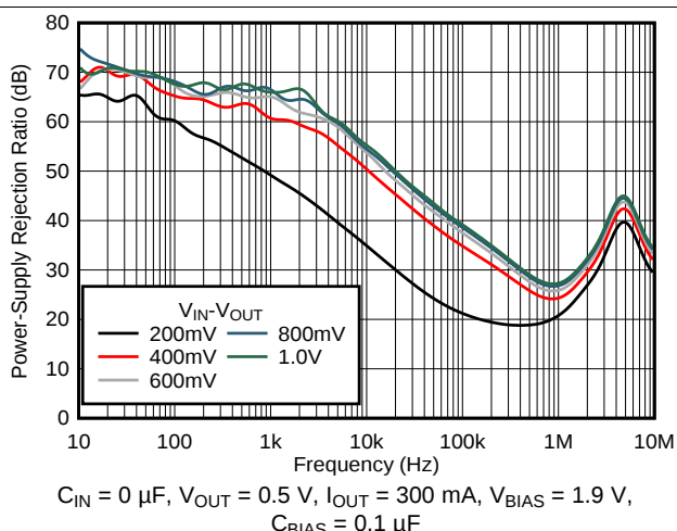
图 30. PSRR vs Frequency and V_{DO}
